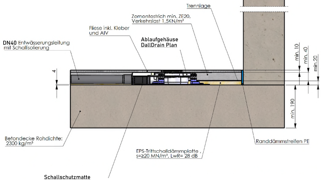
Bild oben: Lage des Prüfaufbaus im Installationsraum (EG vorne).
